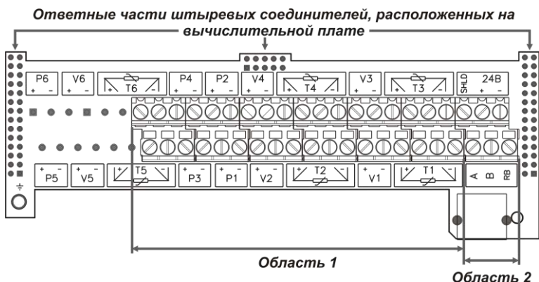
Рисунок Б.2 – Плата подключений вычислителя KARAT-307-4V4T4P
