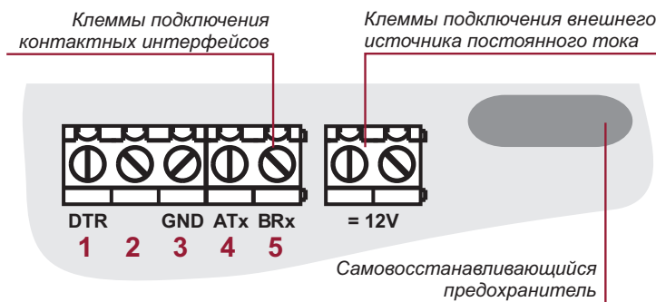
Рисунок 2 – Расположение клеммных соединителей на плате электронного модуля
