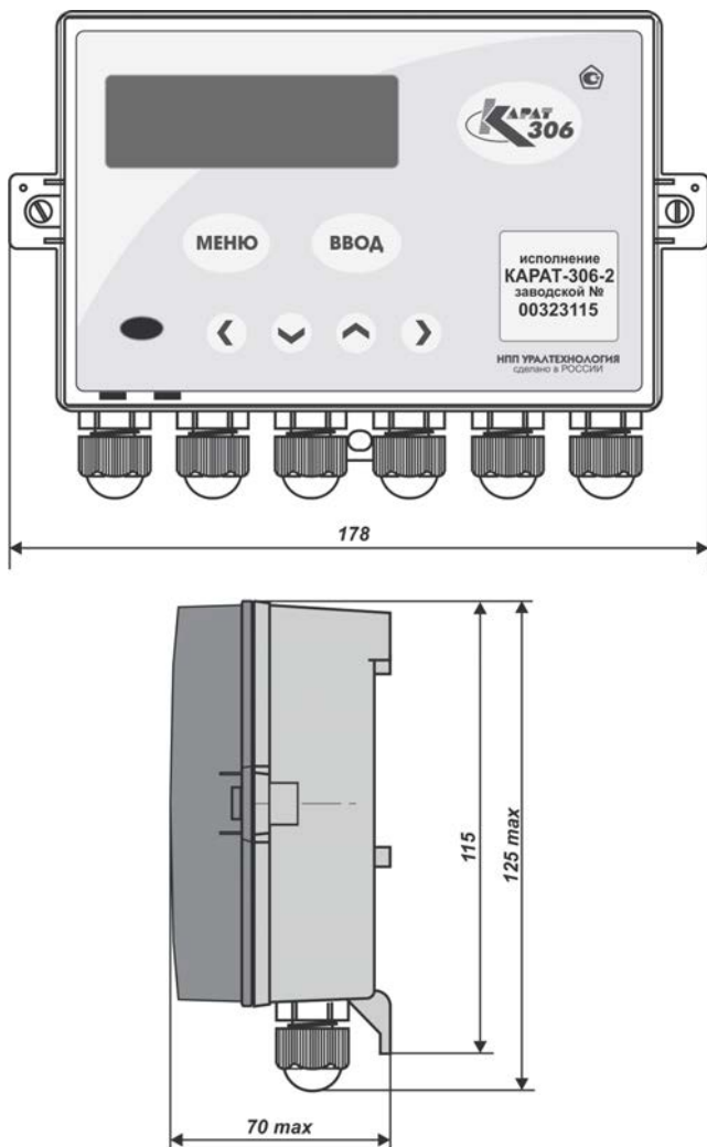
Рисунок А.1 – Габаритные размеры вычислителя КАРАТ-306
